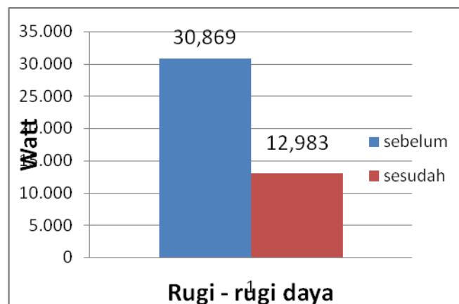
Gambar 1. Grafik Hasil Penyeimbangan Beban Trafo
